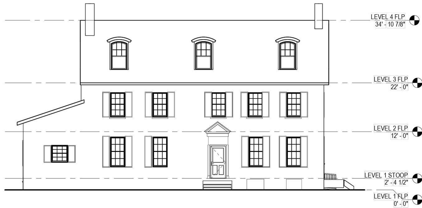
1 EAST ELEVATION A201 SCALE: 1/8" = 1'-0"
