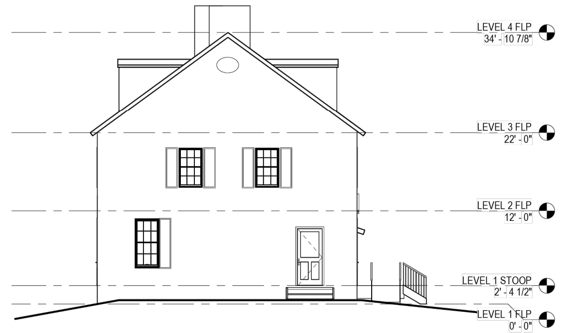
2 NORTH ELEVATION A201 SCALE: 1/8" = 1'-0"
